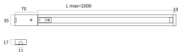
2201-TB-200 (mm)
