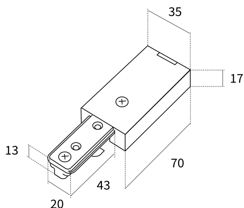
2201-WC-001 (mm)
