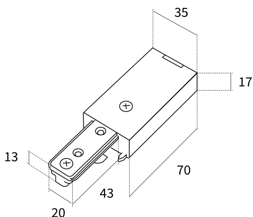
2201-BC-002 (mm)
